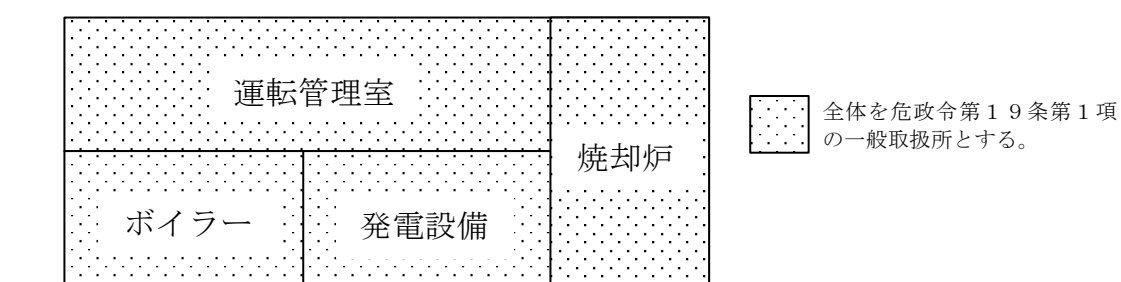
第 8－7 図 全体を一般取扱所とした例
