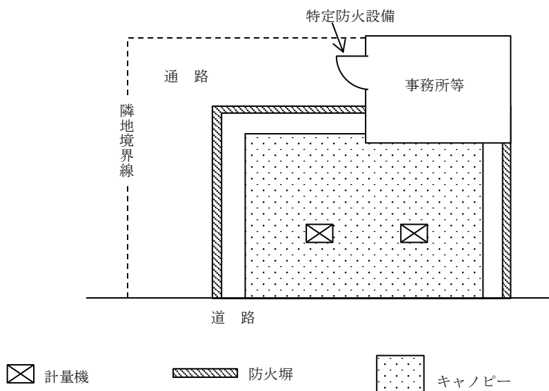
第17-8図 避難口として認められる例
