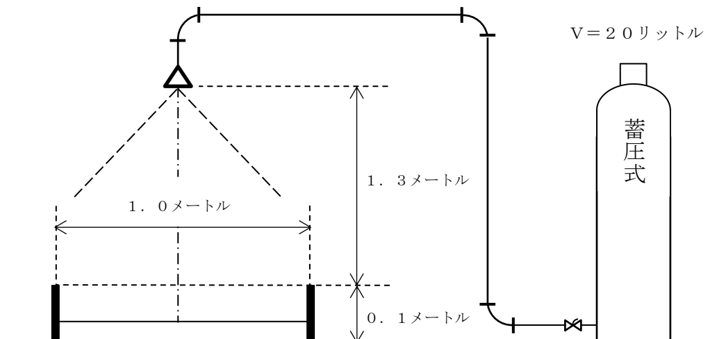
第24-4図 消火試験機材配置図
